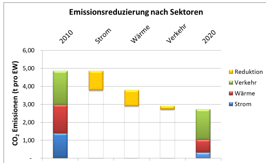
Abbildung 36: Im Diagramm ist die Entwicklung der CO 2 -Emissionen zwischen 2010 und 2020 in den verschiedenen Bereichen dargestellt. Die gelben Balken in der Diagrammmitte zeigen das genaue Ausmaß der Reduktion an CO 2 -Emissionen auf, die in den verschiedenen Bereichen zu erreichen ist.
