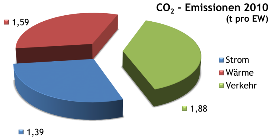
Abbildung 16: Darstellung des CO 2 -Ausstoßes des Hochpustertales im Jahr 2010. Die Werte wurden Tonnen pro Einwohner angegeben.
