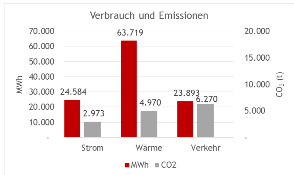
Abbildung 30: In diesem Diagramm sind der Verbrauch und die entsprechenden CO 2 -Emissionen für die drei Bereiche Strom, Wärme und Verkehr für die Gemeinde Toblach dargestellt. Die Daten sind für das Jahr 2010 errechnet worden.
