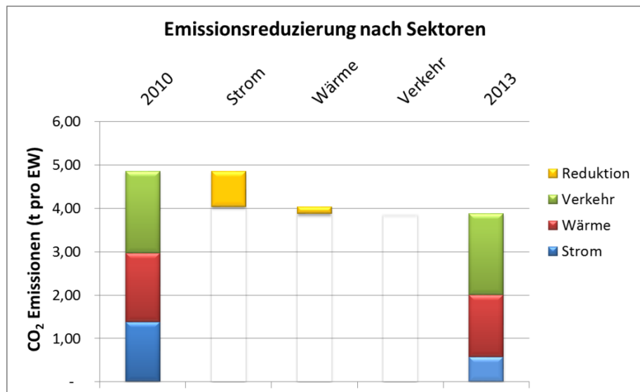
Abbildung 3: Im Vergleich zu 2010 waren die CO 2 -Emissionen in 2013 um 22% geringer. In der Reduktion wurde der größte Beitrag vom Bereich Strom dank einer Zunahme der Produktion aus der Wasserkraft, PV-Anlagen und Fernheizwerken geleistet.
