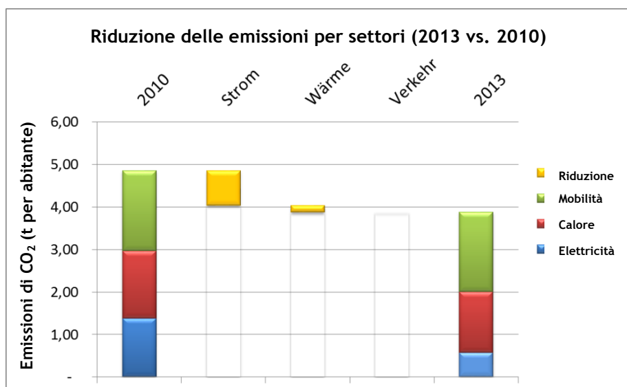
Figura 3: in confronto al 2010, le emissioni di CO 2 dell'anno 2013 erano inferiori del 22%. Nella riduzione il contributo più importante è provenuto dal settore dell'energia elettrica, grazie ad un incremento nella produzione di energia idroelettrica, da impianti fotovoltaici e dagli impianti di cogenerazione del teleriscaldamento.
