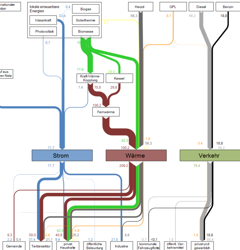
Abbildung 20: In diesem sogenannten „Sankey Diagramm“ werden die Gesamtenergieflüsse (in GWh angegeben) für das Hochpustertal dargestellt. Im oberen Teil ist der Energieverbrauch aus den verschiedenen Energieträgern aufgeteilt und von Pfeilen unterschiedlicher, dem Verbrauchswert entsprechender Größe zum jeweiligen Bereich, bei dem der Verbrauch passiert, geführt.
